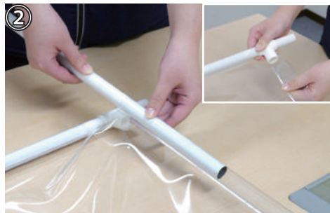
②下段の横パイプを差し込み片側のT型ジョイントに差し込みます
