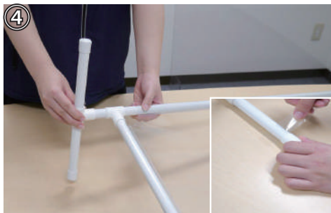
④両サイドにスタンド用パイプをはめ込みテーブルに固定する場合テープをご使用下さい
